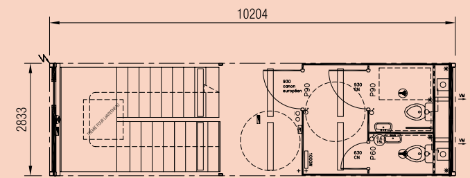
Modul sanitar pt. 20 de persoane și casa scărilor, etaj superior, 30 m 2
