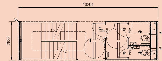
Modul sanitar pt. 20 de persoane și casa scărilor, etaj intermediar, 30 m 2
