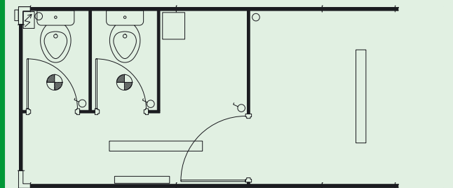
Container Sanitar FR 3015 SD1
