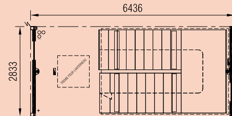
Modul casa scărilor, etaj superior, 19 m 2
