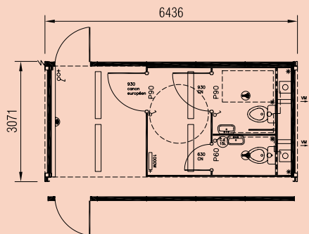
Modul sanitar pt. 20 de persoane, 19 m 2
