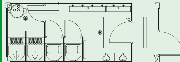
Container Sanitar FR 3015 SC40
