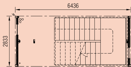
Modul casa scărilor, etaj intermediar, 19 m 2
