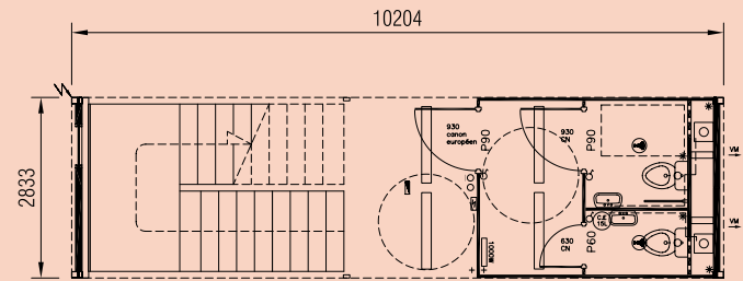
Modul sanitar pt. 20 de persoane și casa scărilor, parter, 30 m 2
